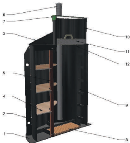
Рисунок 2. Общая схема погреба
